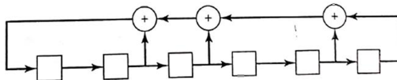
PROBLEM 3-9. Feedback shift register.
